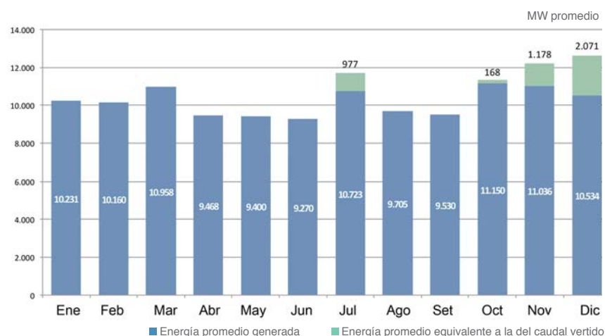
ENERGÍA DISPONIBLE MENSUAL 2015
