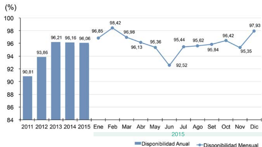
PORCENTAJE DE TIEMPO EN EL PERÍODO CONSIDERADO EN QUE LAS UNIDADES GENERADORAS ESTUVIERON DISPONIBLES PARA OPERACIÓN
